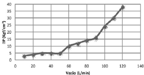
Vazão x Perda de Pressão - CD3269
