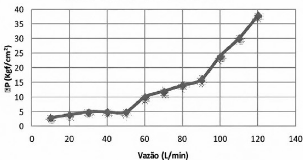
Vazão x Perda de Pressão
